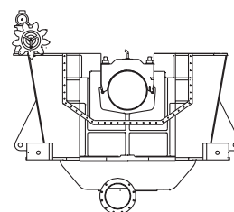
Bedplate section
