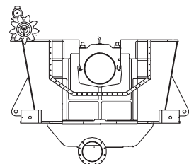
Bedplate section
