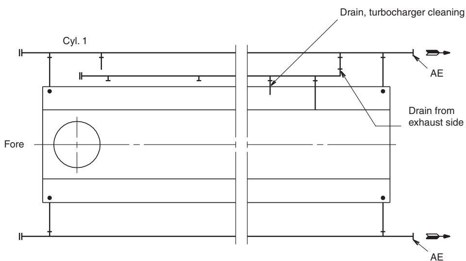
Fig. 8.07.02: Bedplate drain pipes
